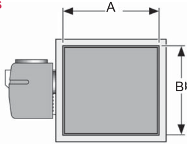
End inlet spigot (HN/HD)
